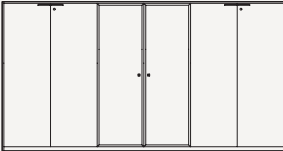
303,6 x 46 H.159,8 cm 119½" x 18" H.63" Armadio mod. A100 A100 Cabinet - Armoire A100 - Schränke A100 - Kasten A100 - Armario A100
