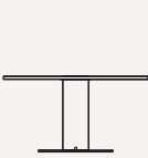
Ø140 H.74 cm Ø55" H.29" Tavolo riunione Meeting table - Table de réunion - Konferenztisch - Vergadertafel - Mesa de reunión
